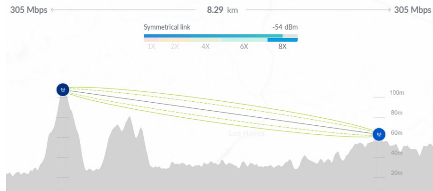
Figura 2. Simulación de enlace Cuajinicuilapa – Punto estratégico
