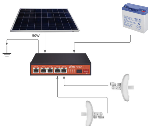
Figura 4. Funcionamiento del switch PoE WI-PS306GF-UPS
